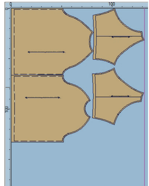
Расположение деталей при раскрое, ширина полотна 180 см
