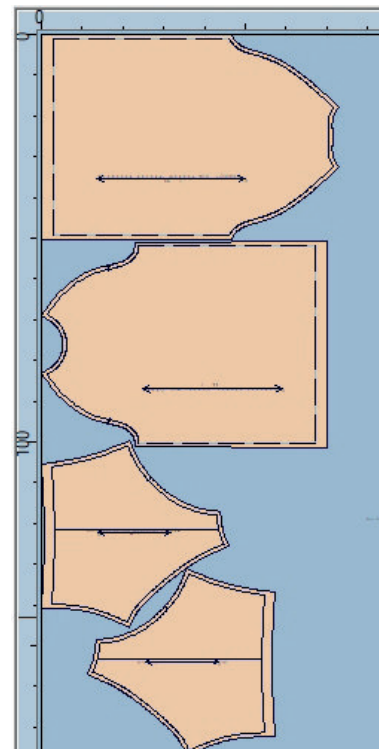
Расположение деталей при раскрое, ширина полотна 180 см
