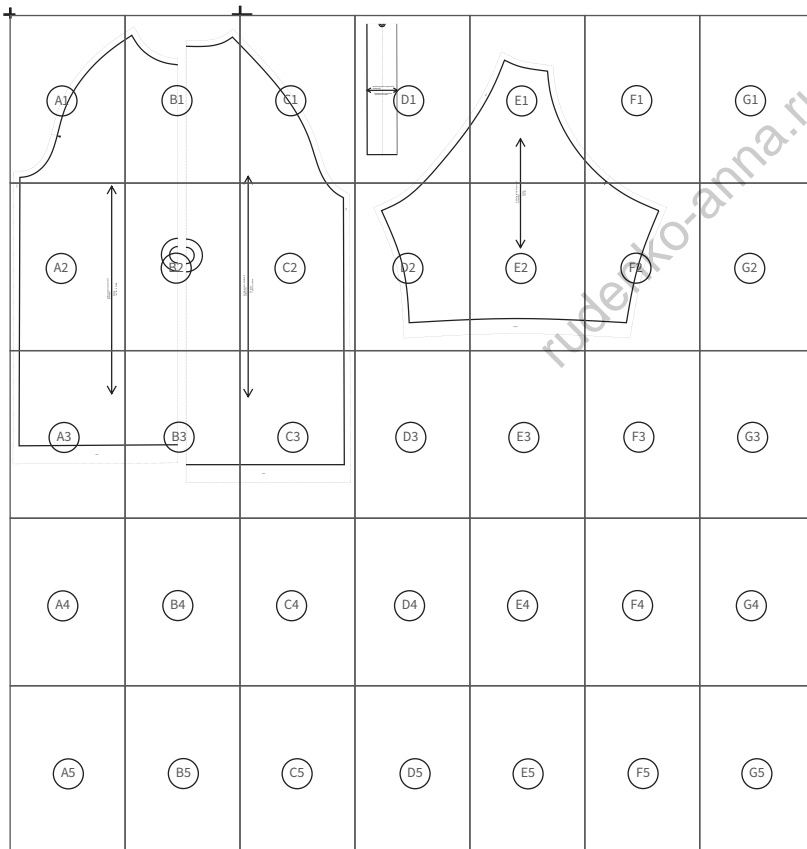
Схема сборки деталей на бумажных листах А4
