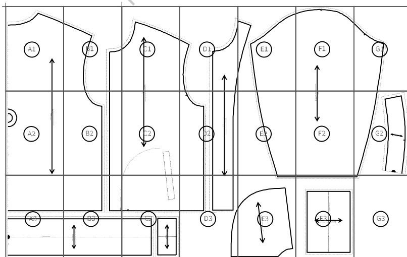
Схема расположения деталей на бумажных листах формата А4
